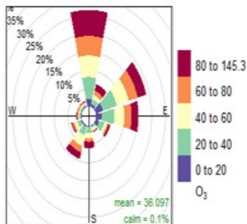
Figura 41- Rosa dos ventos para a EAQA VSL: inverno (A), primavera (B), outono (C), verão (D), concentrações de O_3 em \mu g m^{-3}
