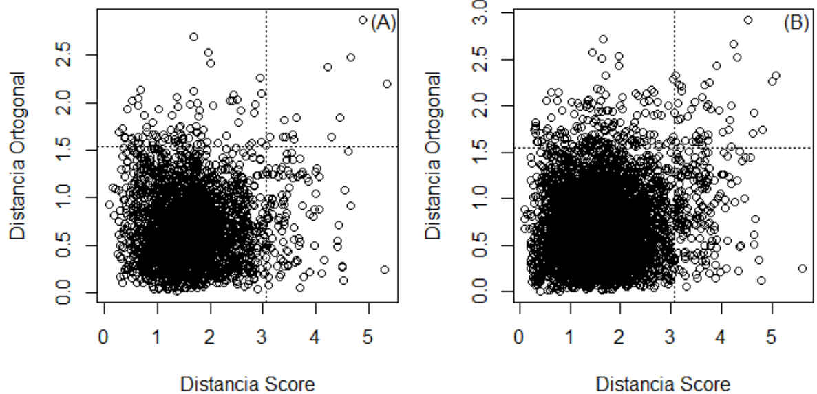
Figura 24- RBOPCA para a EAQA VSL de 2014-2018 para a estação do ano outono: antes da imputação dos dados (A) e após a imputação (B)
