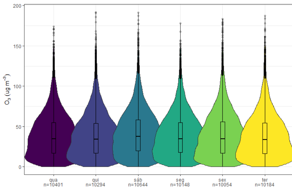
Figura 38- Diagrama violino para os diferentes dias da semana para o O_3 ( \mu g\ m^{-3} )
