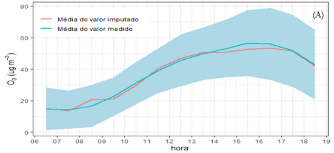
Figura 31 - Comparação entre os valores médios medidos e os valores médios imputados para ADN_out (A), ADN_pri (B), ADN_ver (C), ADN_inv (D)
