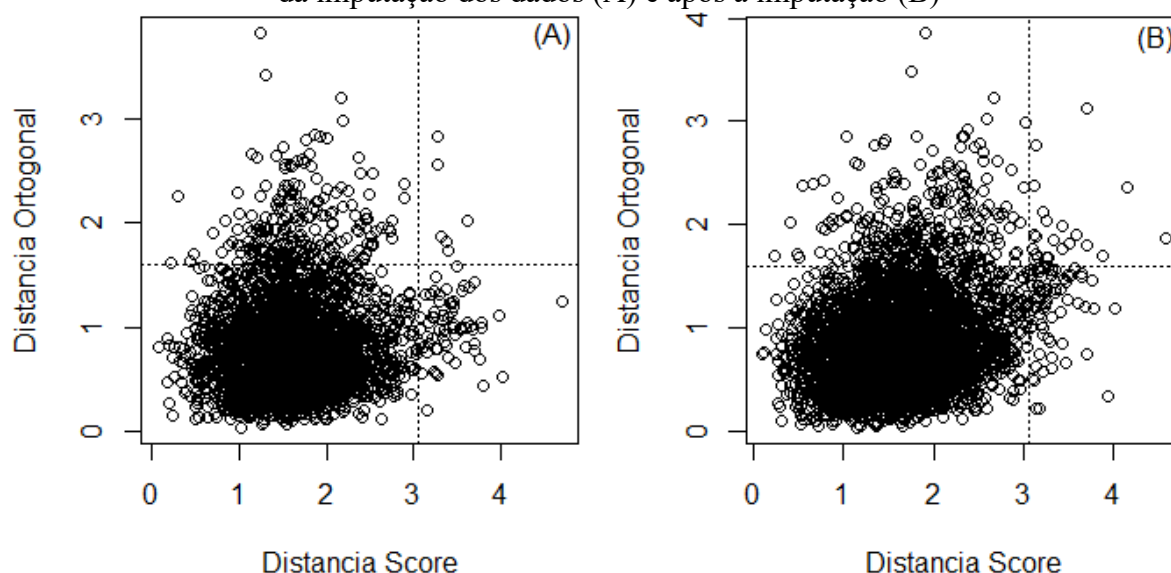
Figura 19- RBOPCA para a EAQA PDC de 2014-2018 para a estação do ano inverno: antes da imputação dos dados (A) e após a imputação (B)
