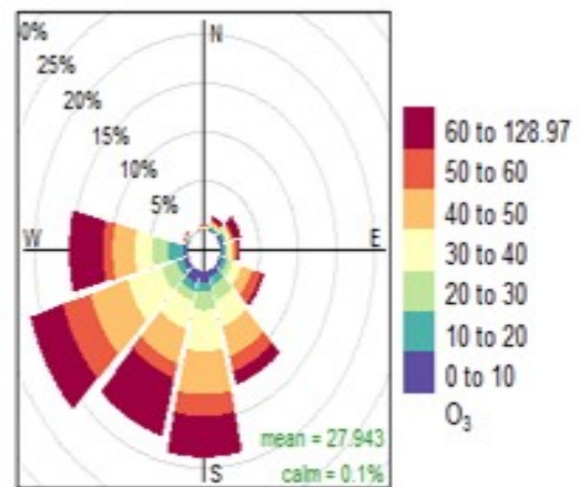
Figura 42- Rosa dos ventos para a EAQA INE: inverno (A), primavera (B), outono (C), verão (D), concentrações de O_3 em \mu g\ m^{-3}
