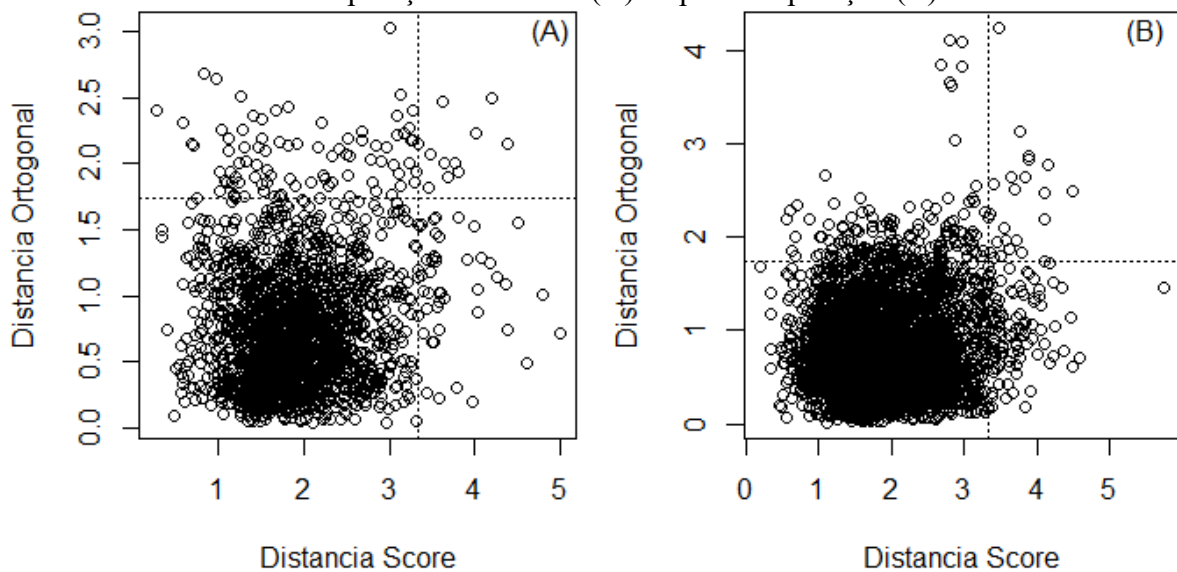
Figura 16- RBOPCA para a EAQA ADN de 2014-2018 para a estação do ano outono: antes da imputação dos dados (A) e após a imputação (B)
