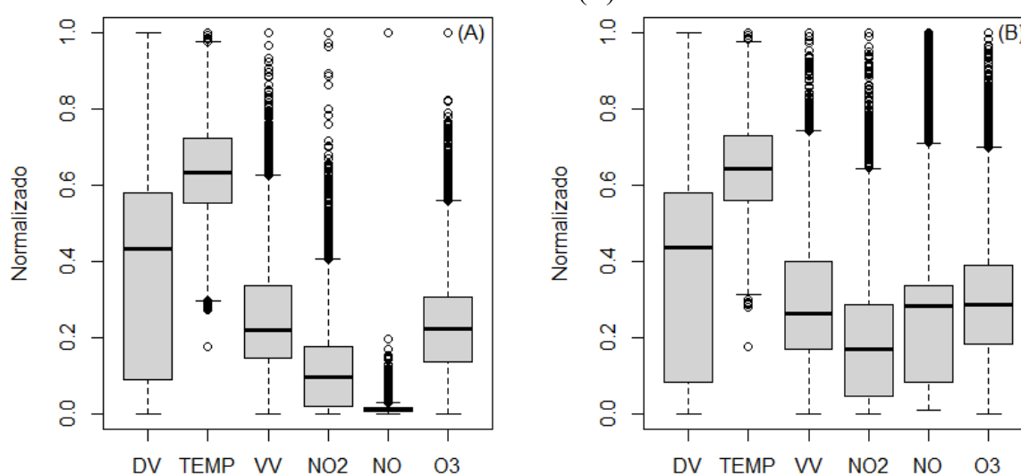
Figura 11- Boxplot normalizado da EAQA de ADN: dados brutos com todas as observações, antes da retirada de pontos anômalos (A) e dados refinados após a retirada de pontos anômalos (B).
