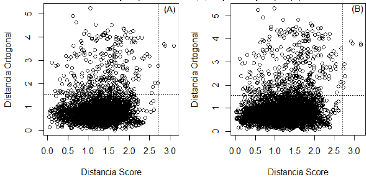
Figura 21- RBOPCA para a EAQA PDC de 2014-2018 para a estação do ano primavera: antes da imputação dos dados (A) e após a imputação (B)
