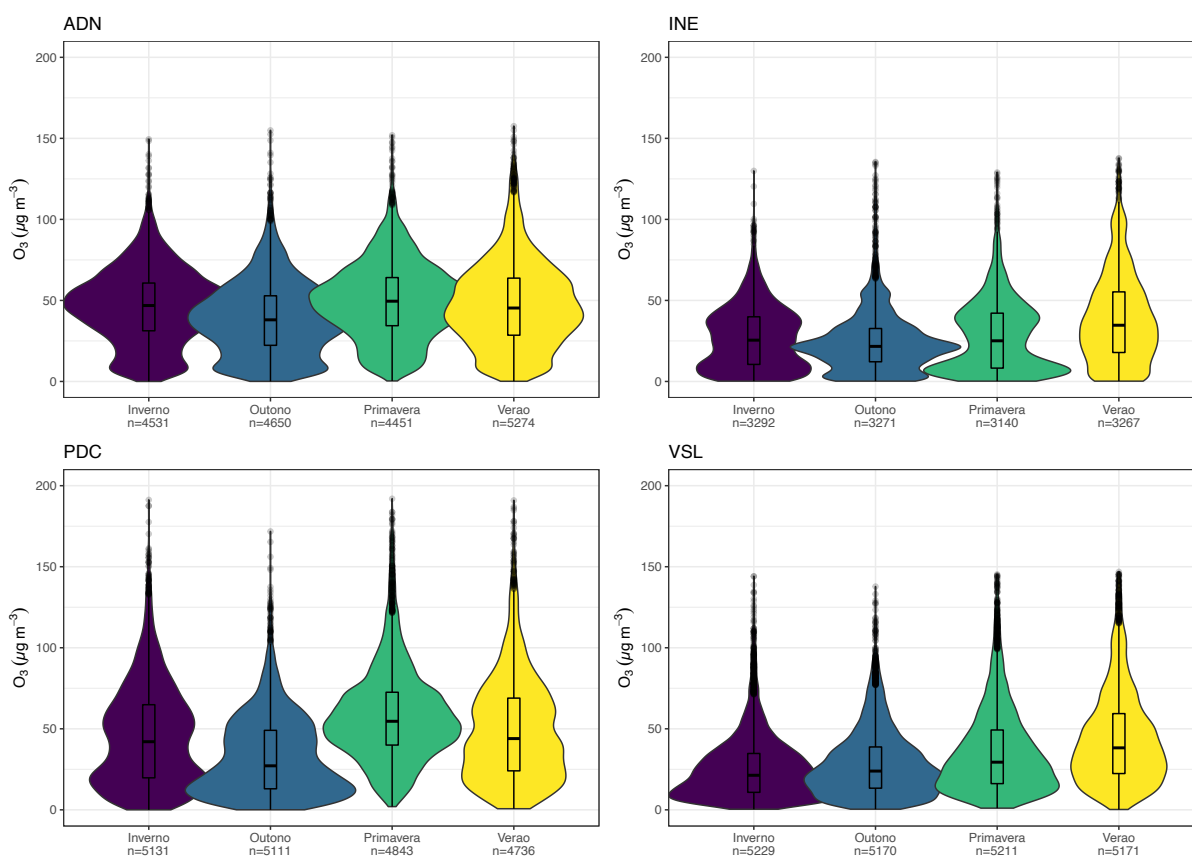
Figura 35- Distribuição por violino para ADN, PDC, VSL e INE para diferentes estações do ano
