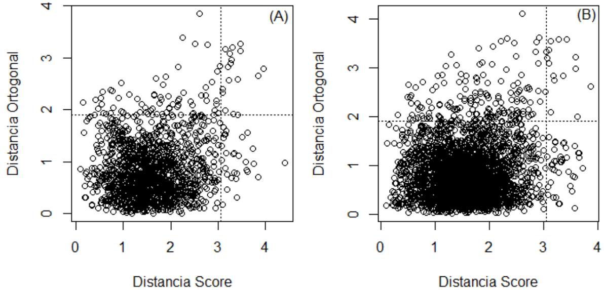
Figura 29- RBOPCA para a EAQA INE de 2014-2018 para a estação do ano primavera: antes da imputação dos dados (A) e após a imputação (B)
