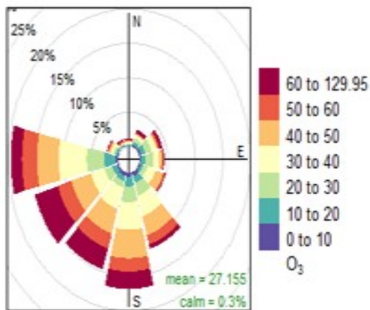
Figura 42- Rosa dos ventos para a EAQA INE: inverno (A), primavera (B), outono (C), verão (D), concentrações de O_3 em \mu g\ m^{-3}
