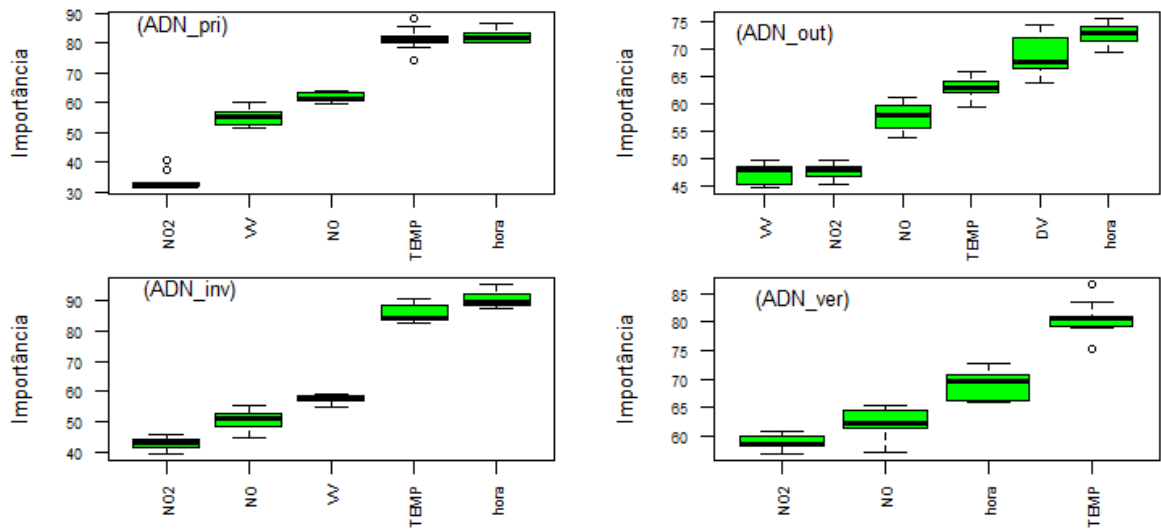
Figura 51- Classificação Boruta para a ADN EAQA
